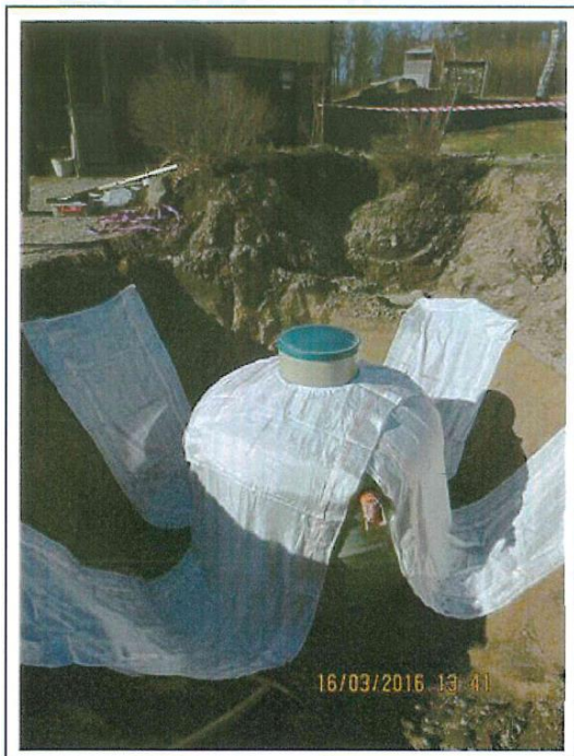
Förankrad med Baga förankringsduk
