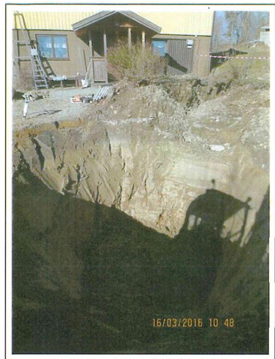
Schaktbotten för slamavskiljare
