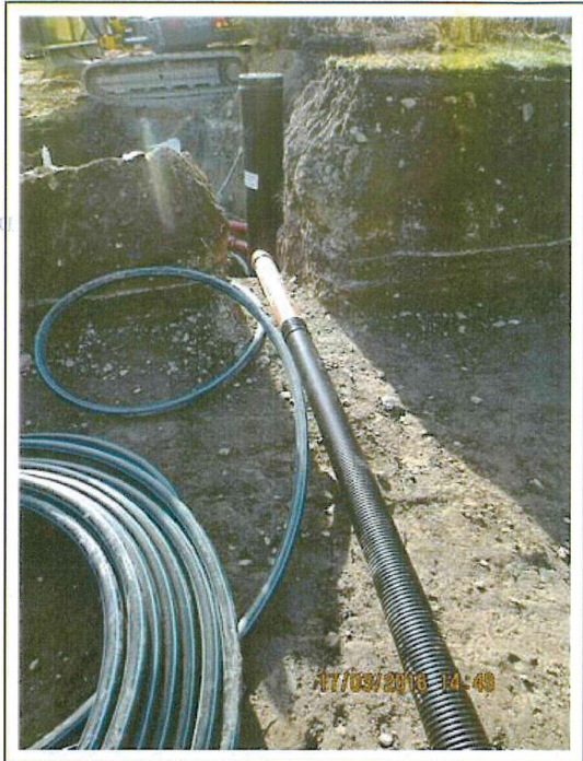
Provtagningsbrunn
