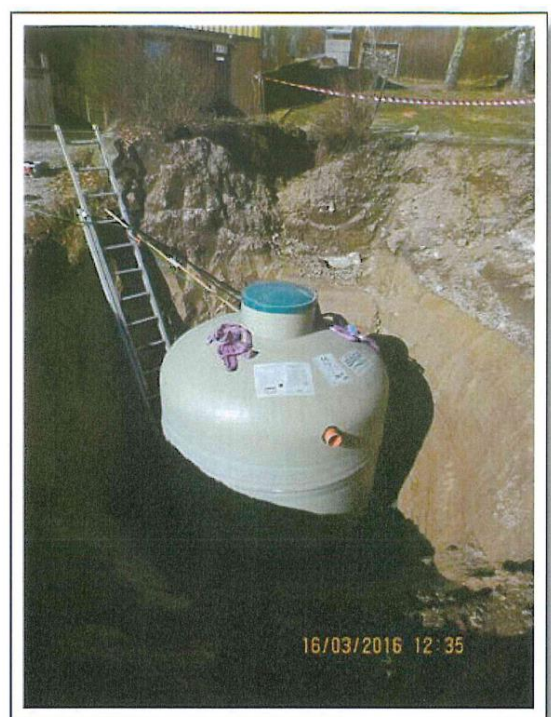
Baga slamavskiljare 4000 liter
